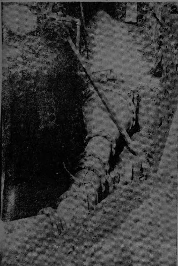
CONCLUIDA LA INSTALACION DE TUBERIA DE PUENTE DE MULAS. Puede apreciarse en esta fotografía la interconexión de la tubería de 36 pulgadas de diámetro procedente de Puente de Mulas, con la tubería de 16 pulgadas de diámetro que abastece los tanques del sur. Se ven el codo, niples y tubería de reducción y parte de la T que permitirá la inyección de agua del nuevo acueducto a los tanques y a la tubería de 16 pulgadas. Se dejó una prevista para conectar tubería de 30 pulgadas de diámetro. El Servicio Nacional de Acueductos y Alcantarillado ejecutó estos trabajos en cuatro horas, tiempo récord. El acueducto de Puente de Mulas va llegando a sus etapas finales y ya se están realizando las pruebas de tubería. Luego se iniciará la prueba de equipos.
